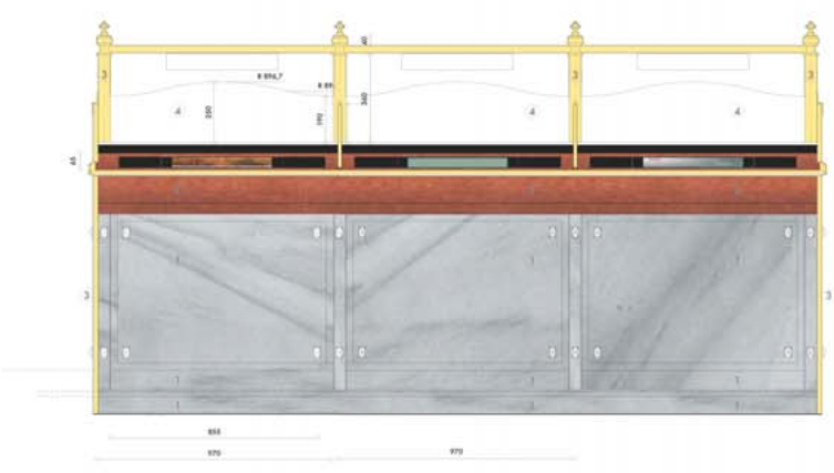
ALZADO LATERAL
