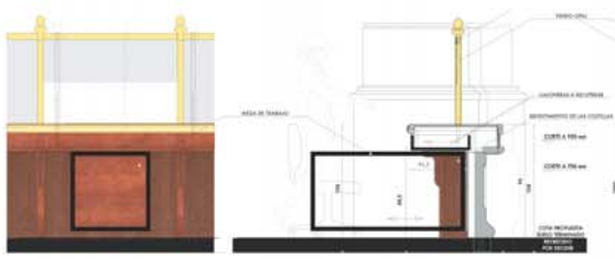
ALZADO LATERAL
