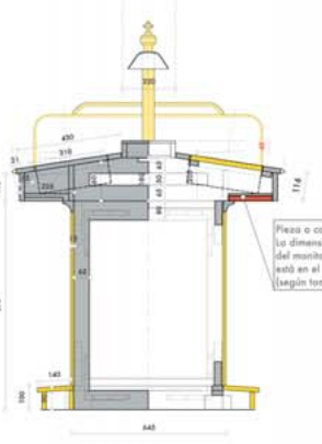
SECCIONES AA/BB
